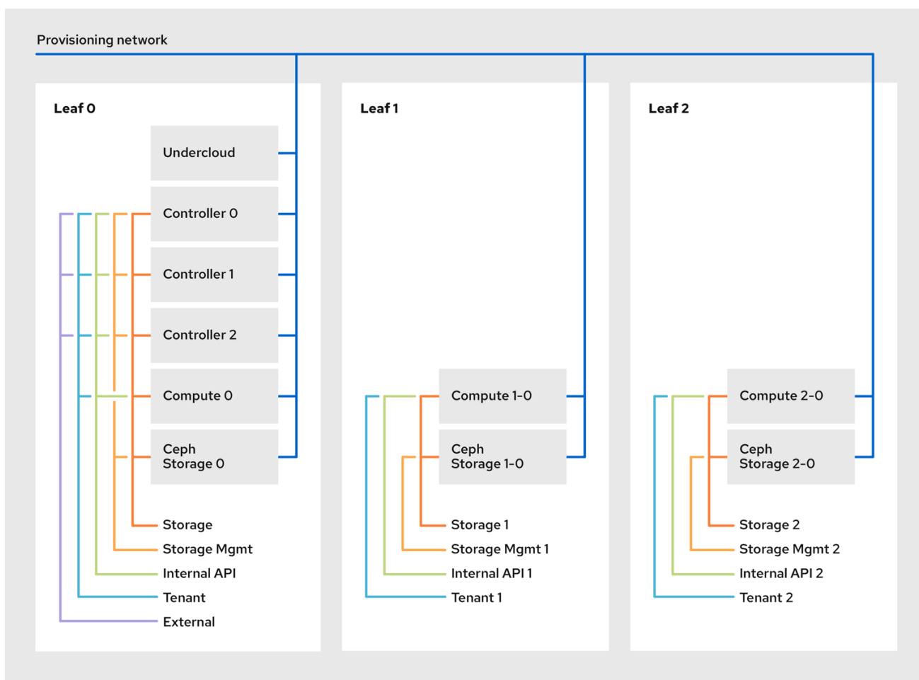
그림 1.2. spine-leaf 네트워크 토폴로지
