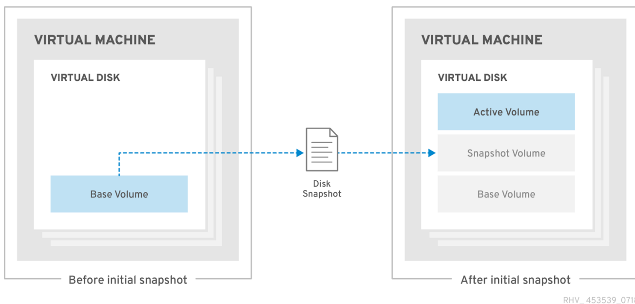
그림 8.1. 초기 스냅샷 생성
