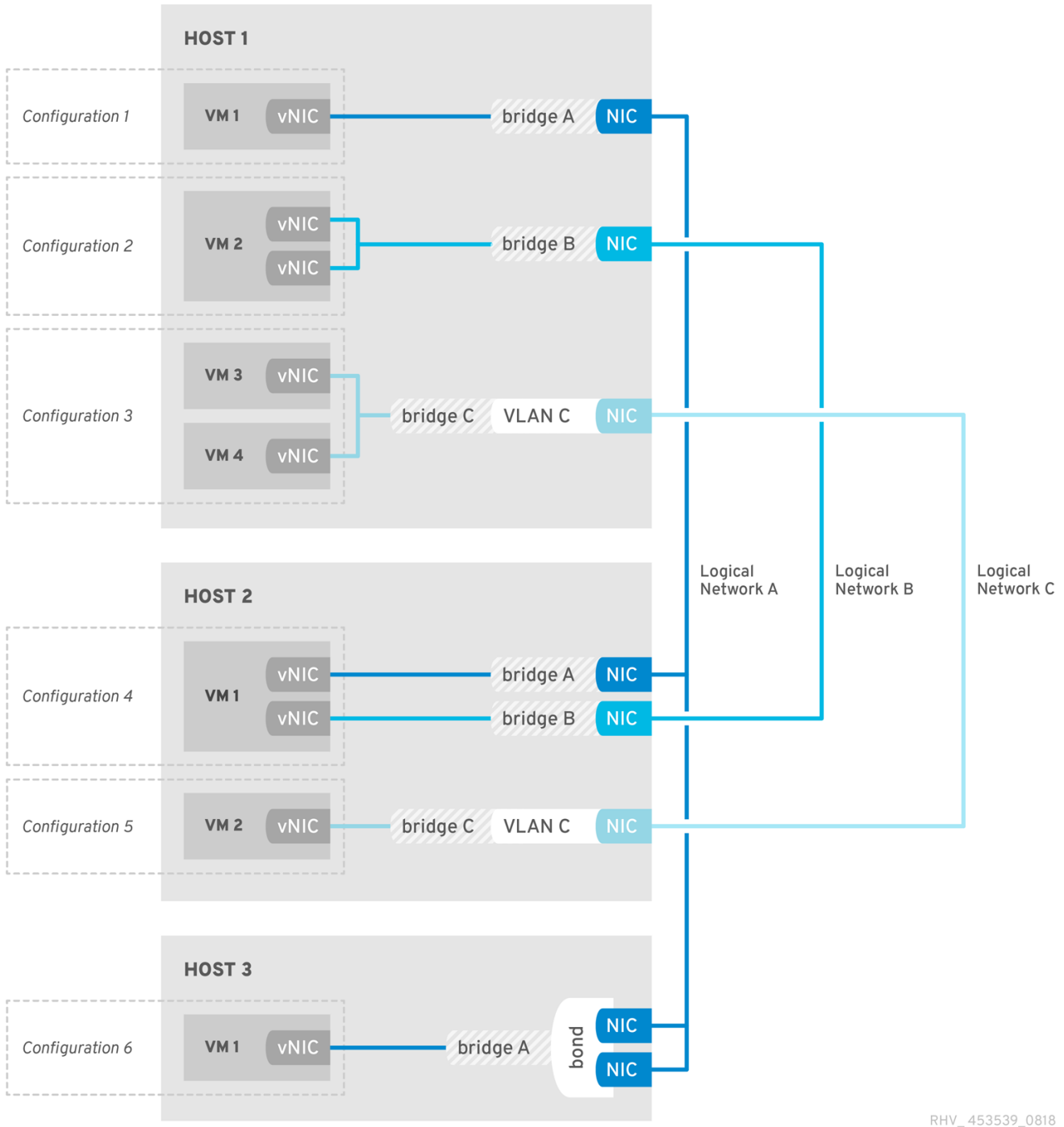
그림 3.1. 클러스터 내의 네트워킹
