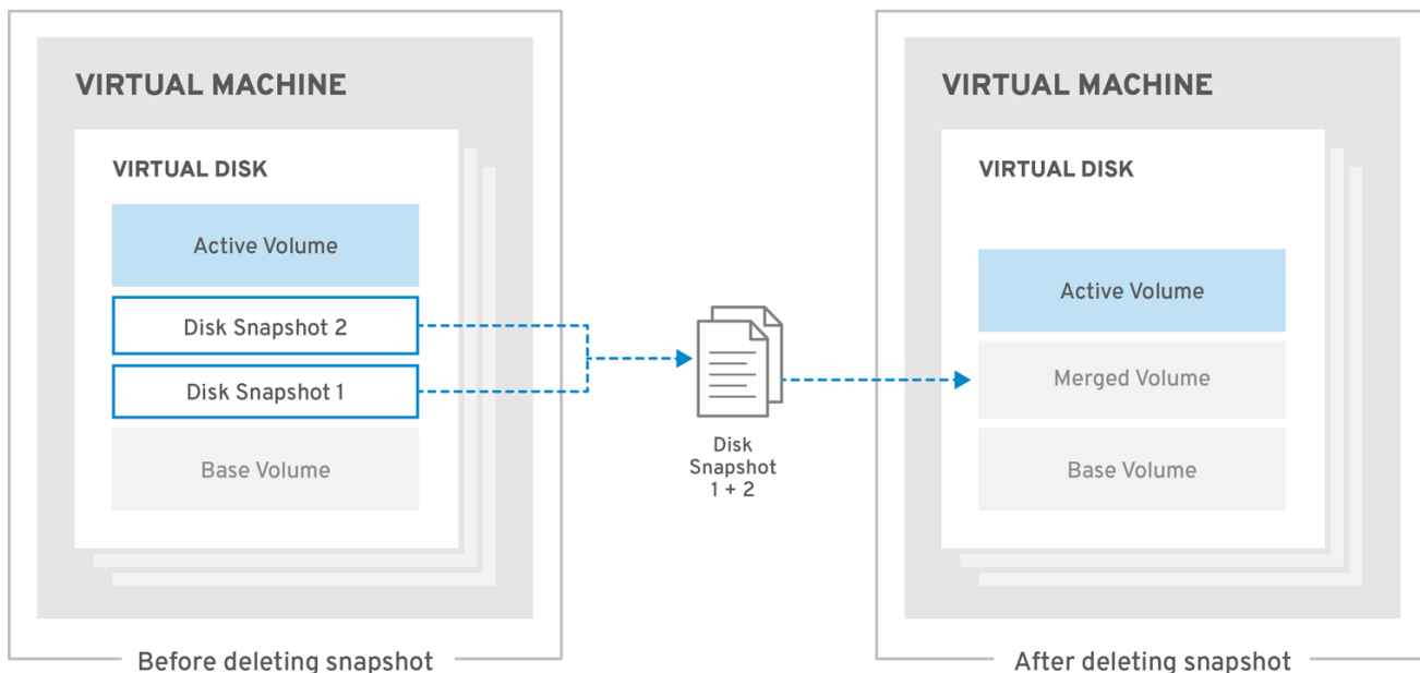
그림 8.4. 스냅샷 삭제
