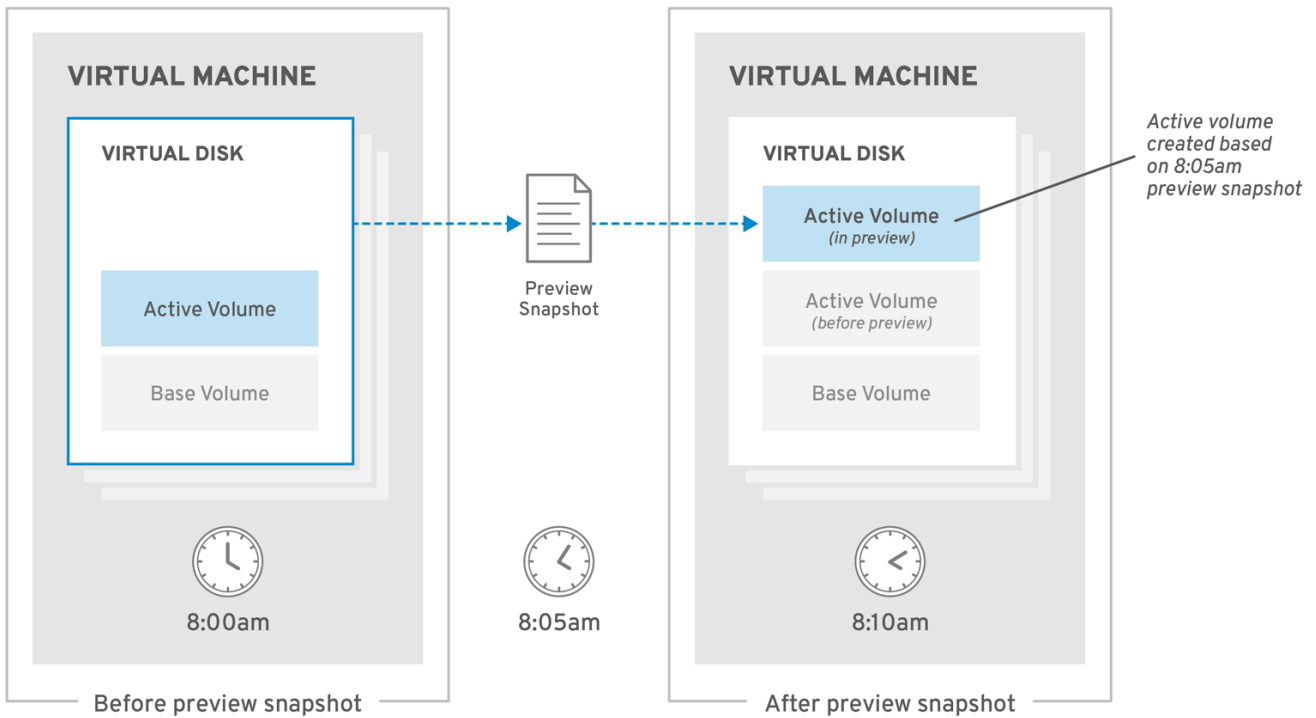
그림 8.3. 스냅샷 프리뷰
