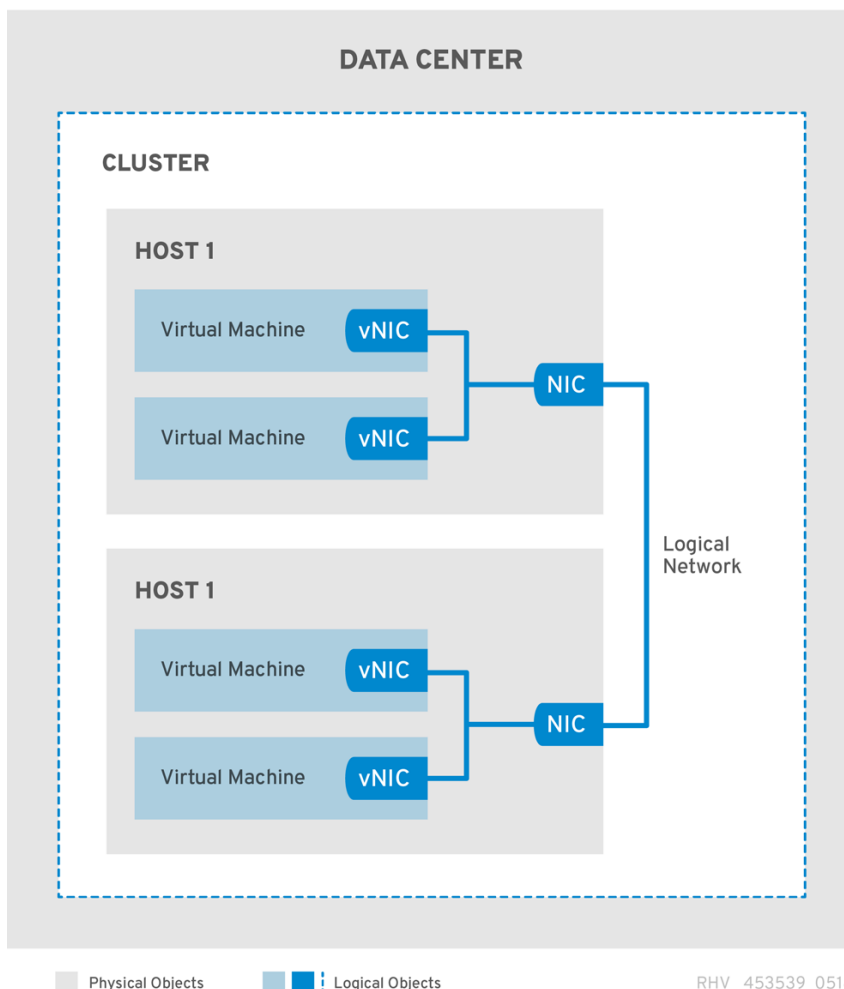
그림 1.3. 네트워크 아키텍처
