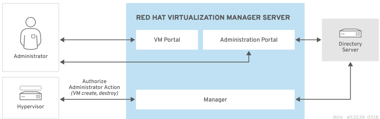
그림 6.1. GSSAPI 인증
