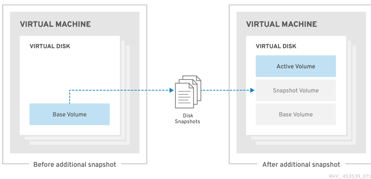
그림 8.2. 추가 스냅샷 생성
