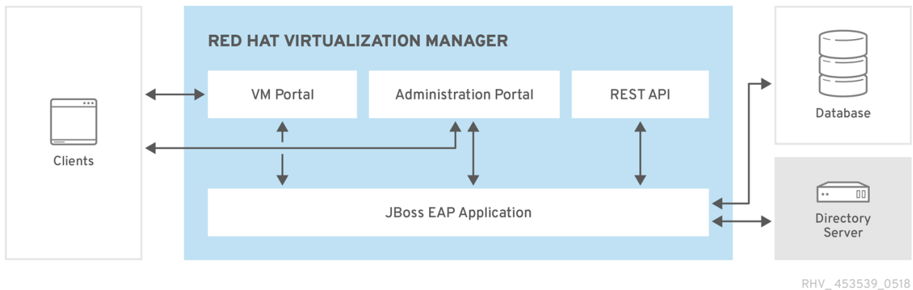
그림 1.1. Red Hat Virtualization Manager 아키텍처
