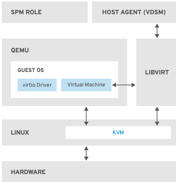
그림 1.2. 호스트 아키텍처
